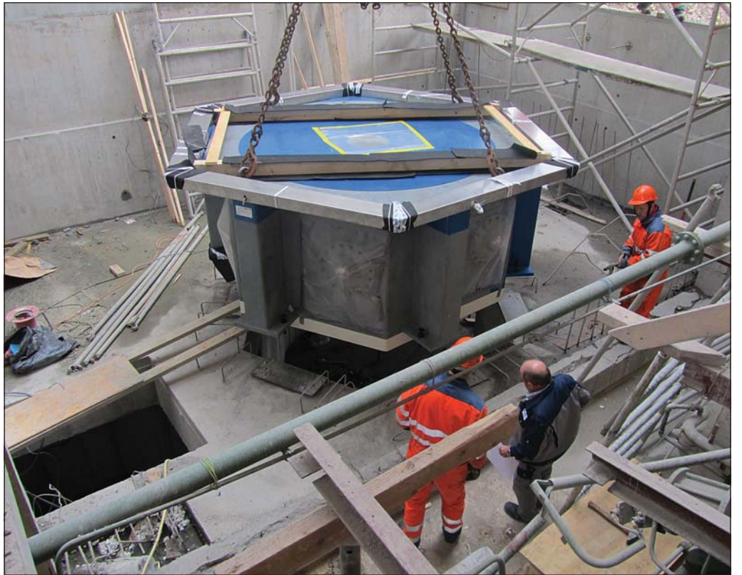
Nýja túrbínin var hífð inn í stöðvarhús Mjólkárveikjunnar. Ljós: Steinar R. Jónasson.
