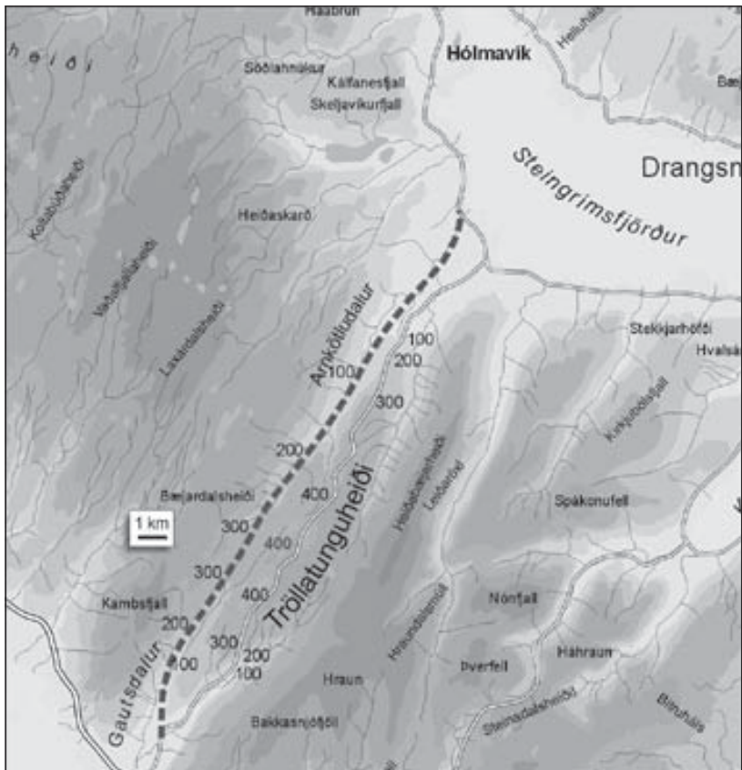
Kort af fyrirhuguðu vegstæði um Arnkötludal og Gautsdal. Mynd: leið.is
