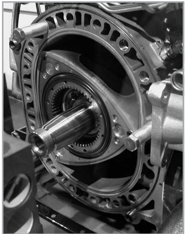
Séð inn í sundurtekinn Wankel-mótor.
